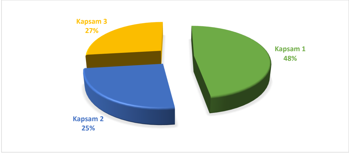
Şekil 7. 2017 Yılı Karbon Emisyonlarının Kapsamlara Göre Dağılım Grafiği
