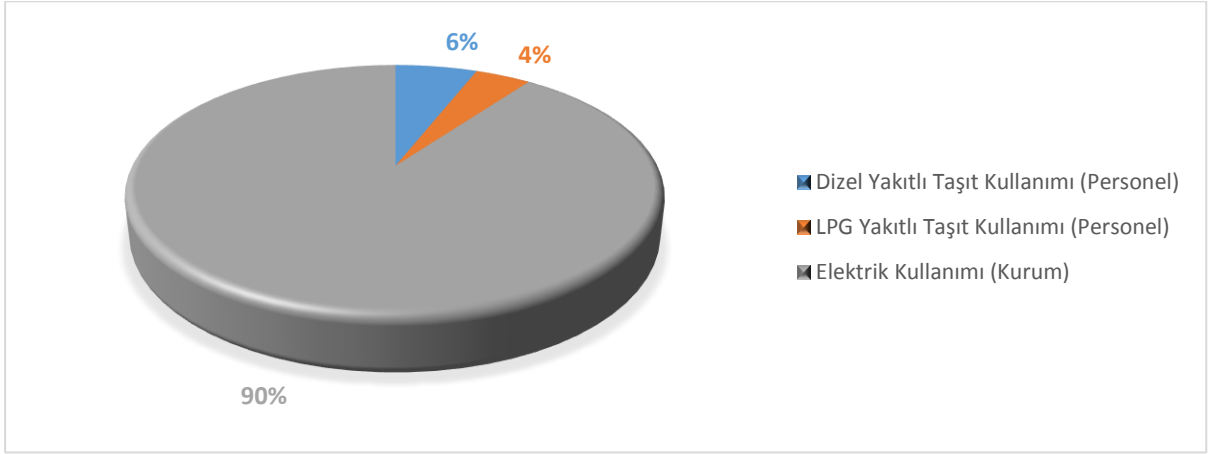
Şekil 9. Kapsam 3 Emisyonlarının Dağılımı
