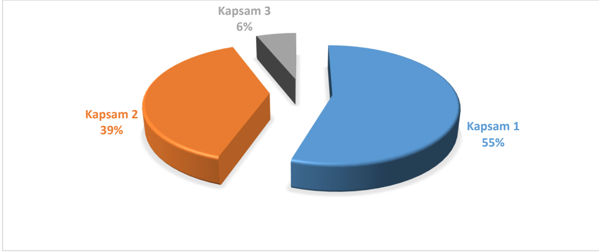
Şekil 7. 2017 Yılı Karbon Emisyonlarının Kapsamlara Göre Dağılım Grafiği
