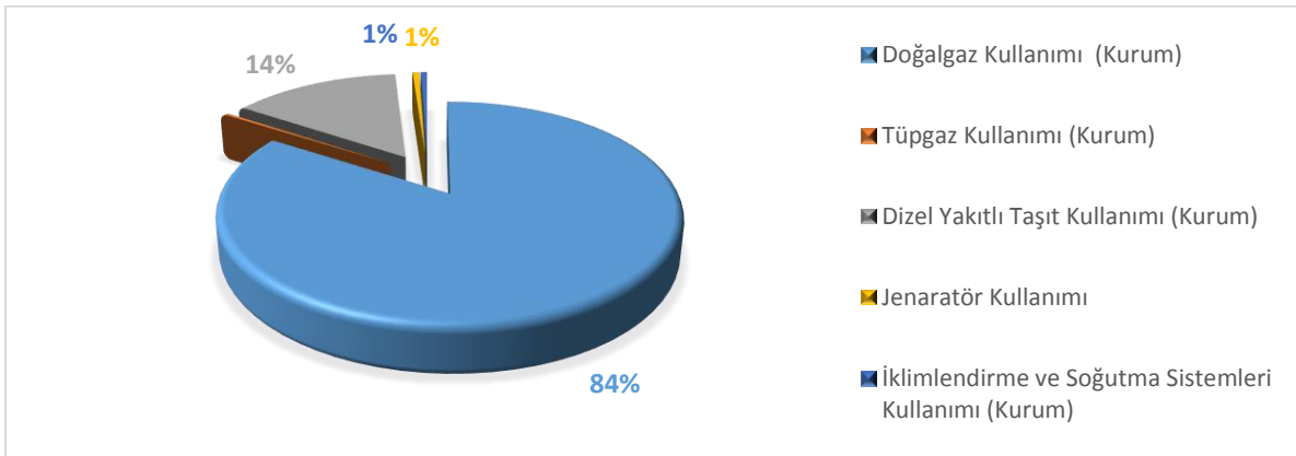
Şekil 8. Kapsam 1 Emisyonlarının Dağılımı
